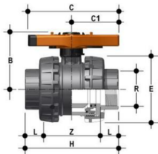
Шаровой кран общего применения VXE ХПВХ с резьбовыми окончаниями, DN65-100 R3" (DN80)
