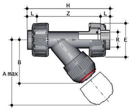
Грязевый фильтр RVUFT PBX с резьбовыми окончаниями, EPDM, FIP R1¼" (DN32)
