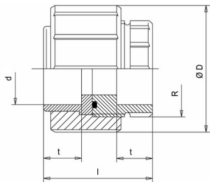
Муфта разборная ПВДФ (Simona) d40 SDR21 PN16
