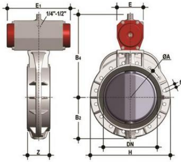
Дисковый затвор промышленного применения FK ПВХ с пневмоприводом, FKM, FIP d16" (DN400)
