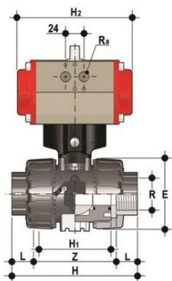
Шаровой кран VKD с пневмоприводом H3 с резьбовыми окончаниями (уплотнение FKM) PP-H R2" (DN50)
