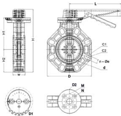
Затвор дисковый с рукояткой PP-H IPS d90 (DN80)
