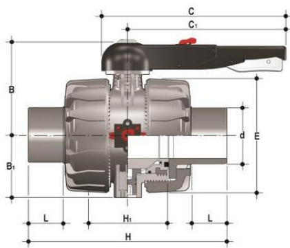
Шаровой кран промышленного применения VKD ХПВХ с втулочными окончаниями, DN65-100 d75 (DN65)
