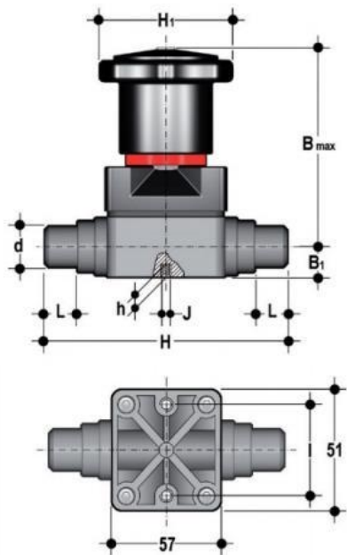
Компактный мембранный клапан СМ ПВХФ с втулочными окончаниями d20 (DN15)
