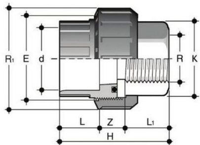
Муфта разборная переходная ХПВХ/ нержавеющая сталь ВР 50х1 1/2" PN16
