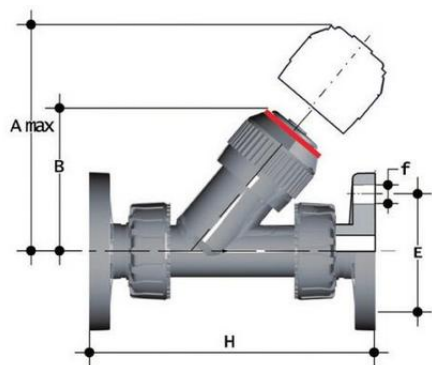
Угловой обратный клапан VR с фланцевыми окончаниями, (уплотнение FKM) PP-H d90
