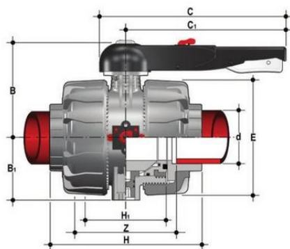
Шаровой кран промышленного применения VKD С муфтовыми окончаниями (уплотнение EPDM) PP-H d75
