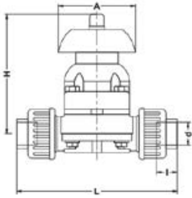
Мембранный клапан IDK ПВХ с муфтовыми окончаниями, PTFE, IPS d75 (DN65)
