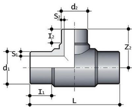
Тройник редукционный для стыковой сварки PP-H FIP 110x63 SDR17.6 PN10
