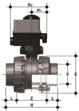
Шаровой кран VXE ПВХ с пневмоприводом, EPDM, FIP d110 (DN90)
