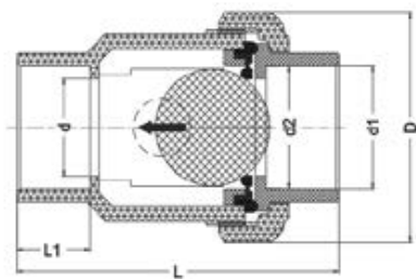
Обратный клапан шаровой с одним разборным соединением, муфтовые окончания PP-H IPS d90 (DN80)
