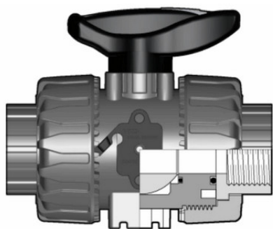
Шаровой кран промышленного применения VKD ХПВХ с муфтовыми окончаниями d32 (DN25)
