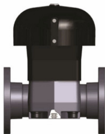
Мембранный клапан VM PBX с пневмоприводом ДвД, фланцевые окончания, FKM, FIP d110 (DN100)
