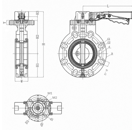
Затвор дисковый в корпусе FRPP (диск - НПВХ) с рукояткой промышленного применения FKM IPS 90 (DN80)
