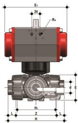
3-х ходовой шаровой кран ТКД ПБХ с пневмоприводом, Т-шар, FIP d32 (DN25)
