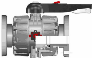
Шаровой кран промышленного применения VKD ХПВХ с фланцевыми окончаниями, DN65-100 d110 (DN90)
