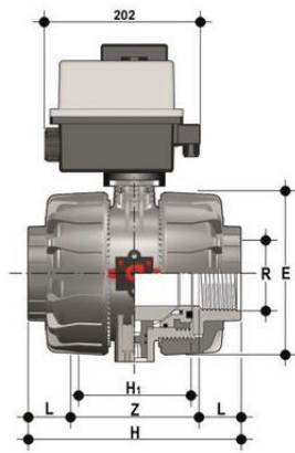
Шаровой кран VKD ПВХ с эл.приводом 90-240V, резьбовые окончания, FKM, FIP R4'' (DN90)
