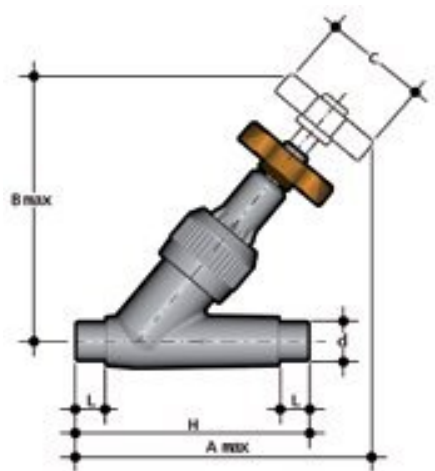
Угловой вентиль VVDV PBX с втулочными окончаниями, EPDM, FIP d16 (DN10)
