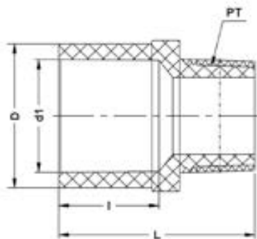
Муфта с НР ХПВХ IPS 75x2½" PN16
