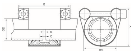
Соединительная муфта GRIP Ø25.0-48.3, NBR, W5 d38
