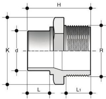
Втулка переходная с НР ПВХ FIP 25x1
