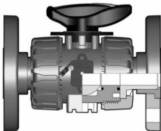
Шаровой кран для регулирования потока VKR ПВДФ с фланцевыми окончаниями d40 (DN32)
