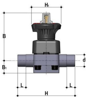
Мембранный клапан DK/L ХПВХ с втулочными окончаниями d25
