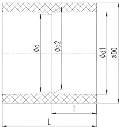
Муфта соединительная ПВХ IPS d40
