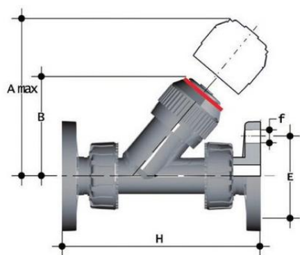
Угловой обратный клапан VR с фланцевыми окончаниями, (уплотнение FKM) PP-H d90 (DN80)
