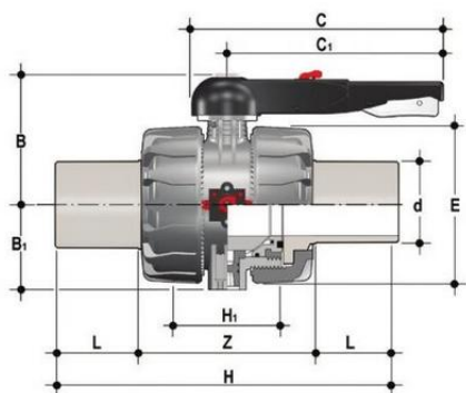
Шаровой кран VKD ПВДФ с длинными патрубками, DN65-110 d110 (DN100)
