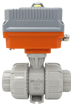
Шаровой кран IVKD ПП-гомополимер с эл.приводом 24V DC, муфтовые окончания, EPDM, IPS d40 (DN32)
