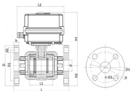
Шаровой кран IVKD ХПВХ с эл.приводом 220V AC, фланцевые окончания d110 (DN100)
