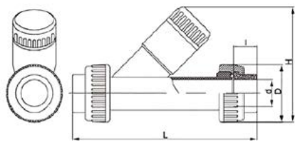
Фильтр сетчатый (грязевой) PP-H IPS d75 (DN65)
