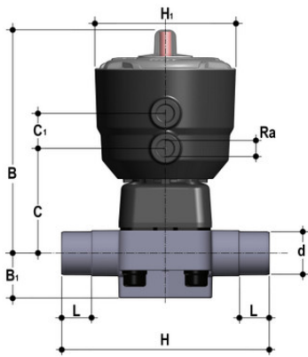
Мембранный клапан ДК ПВХ с пневмоприводом, PN10, втулочные окончания, FKM, FIP d50 (DN40)
