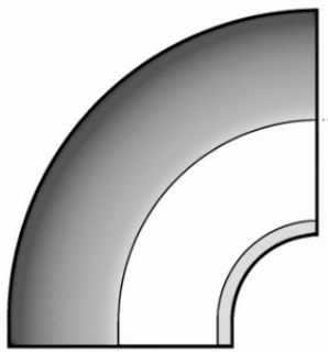
Отвод 90° для стыковой сварки PP-H FIP d500 SDR11 PN6
