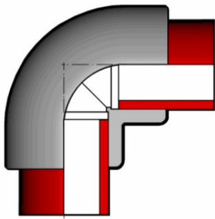
Отвод 90° для раструбной сварки PP-H FIP d40 PN10
