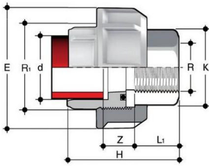
Муфта переходная разборная ВР ПВДФ 63x2 SDR21 PN16
