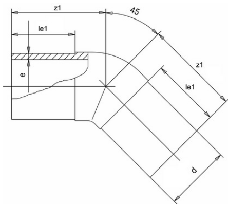
Отвод ПВХ 45° (Simona) d90 SDR21 PN16
