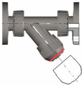
Грязевой фильтр RVUOM с фланцевыми окончаниями (уплотнение EPDM) PP-H d63 (DN50)
