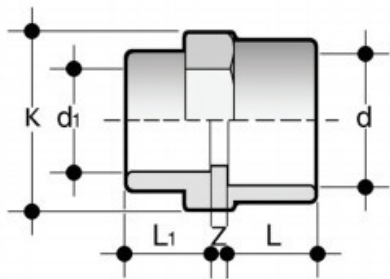
Муфта редукционная ПВХ FIP 110x090
