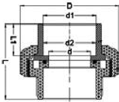
Муфта ХПВХ IPS d25 PN16
