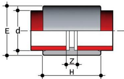
Муфта соединительная ПВХ d20 SDR21 PN16
