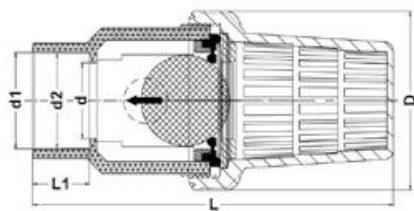
Донный клапан IVZ ПВХ с муфтовыми окончаниями, FKM, FIP d40 (DN32)
