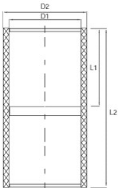
Муфта соединительная ХПВХ IPS (Model A) d40 PN16
