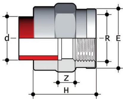
Переходная муфта с ВР, раструбная сварка РР-Н FIP 50x1 1/2 PN10
