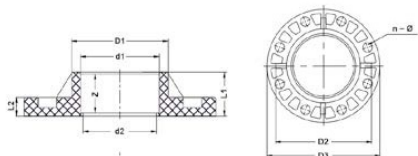
Жесткий фланец ХПВХ IPS (Model B) d315 PN10
