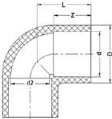
Отвод 90° ХПВХ IPS (Model B) d500 PN10
