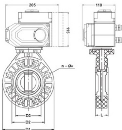
Дисковый затвор IFK ПВДФ с электрическим приводом 220V AC, EPDM, IPS d225 (DN200)
