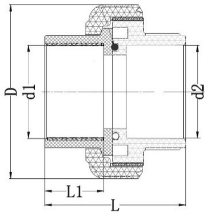
Муфта разборная с ВР, РР-Н IPS d40 PN10
