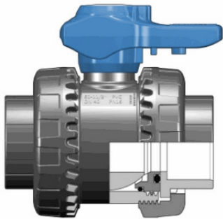
Шаровой кран ПВХ общего применения VEE; муфтовые окончания, EPDM, PIP d25 (DN20)
